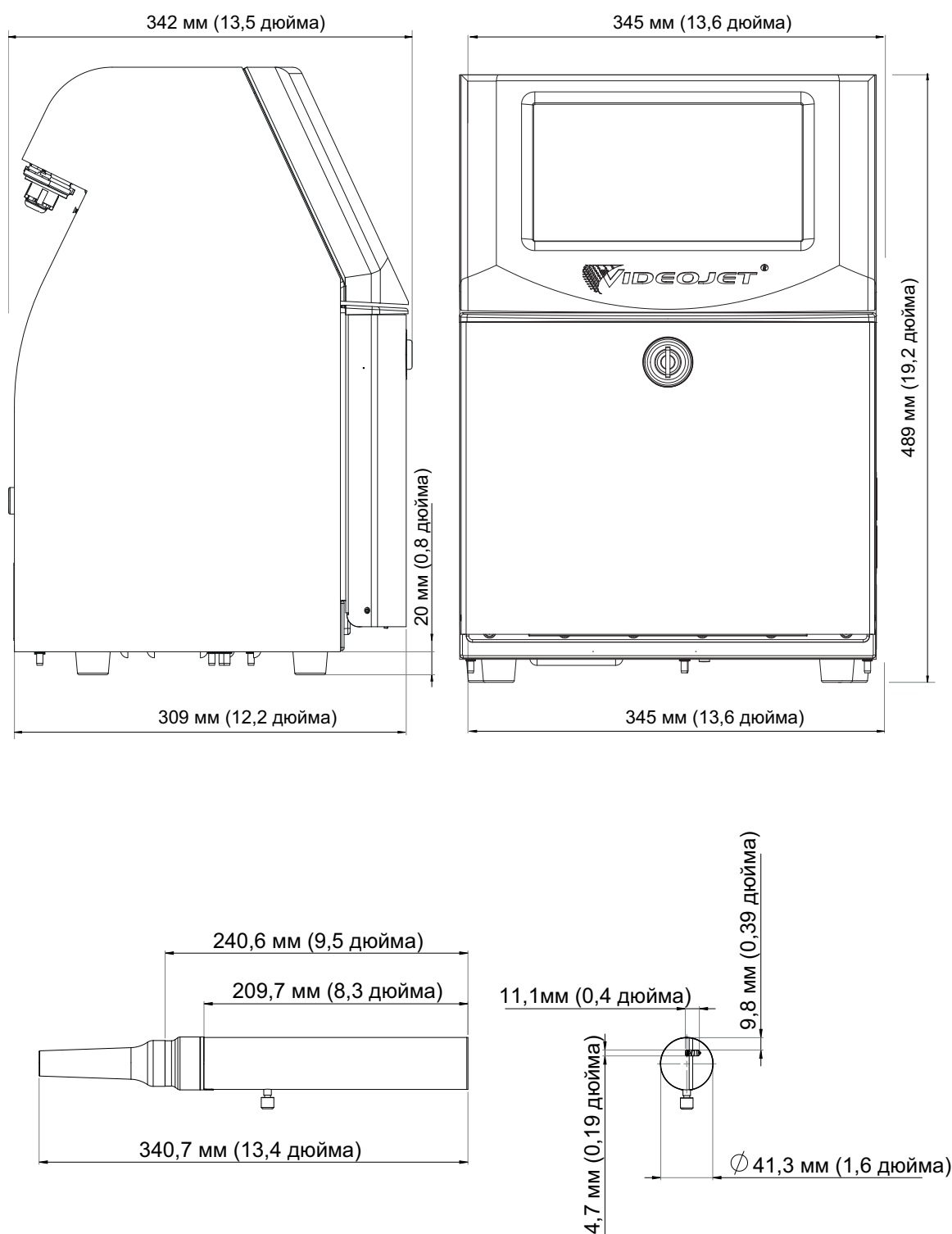
Рис. А-1: Размеры принтера (Videojet 1240/Videojet 1280)
