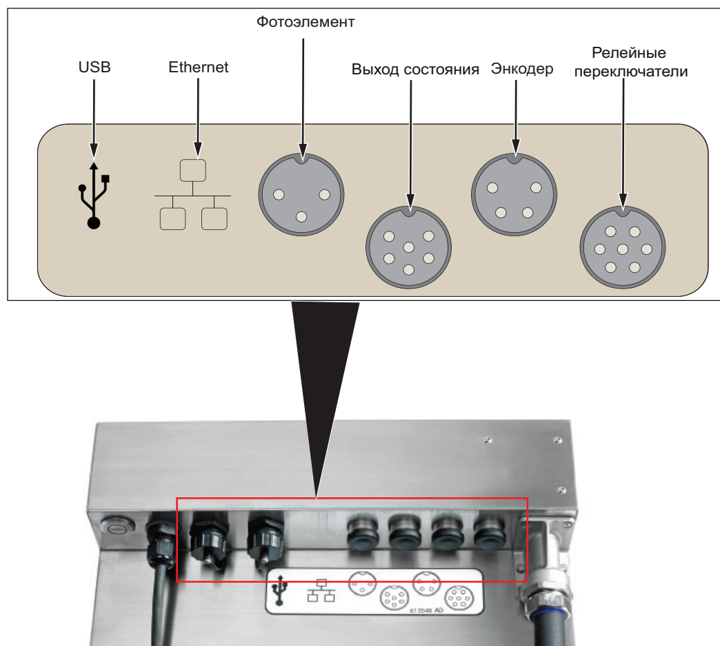
Рис. 3-11: Стандартные разъемы ввода-вывода
