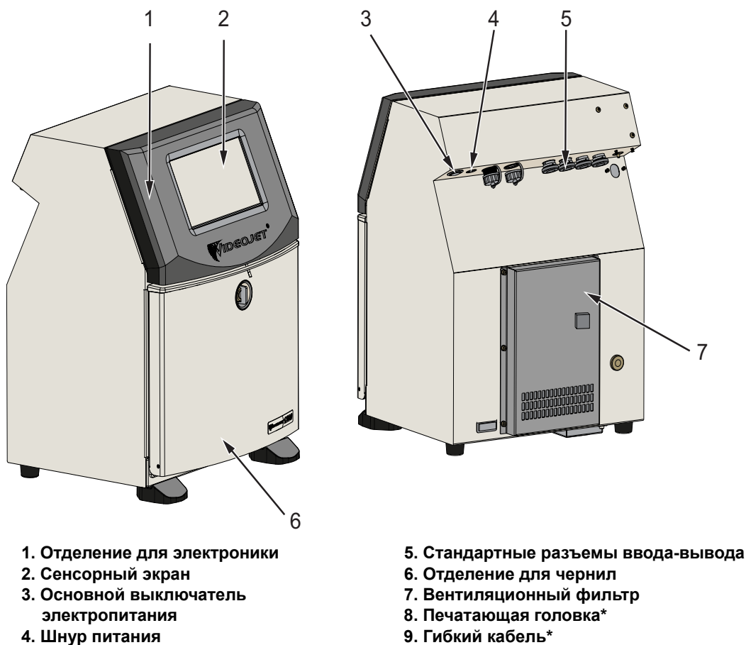
Рис. 3-2: Принтер Videojet 1240/1280
