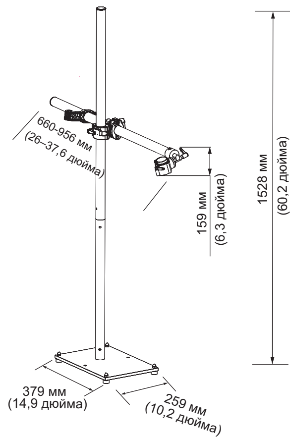
Рис. А-3: Подставка для печатающей головки
