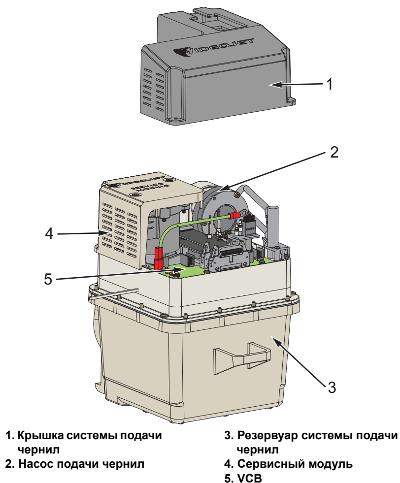
Рис. 3-10: Система подачи чернил
