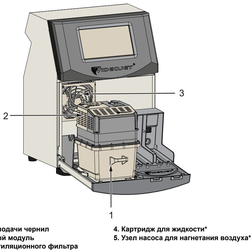
Рис. 3-6: Отделение для чернил
