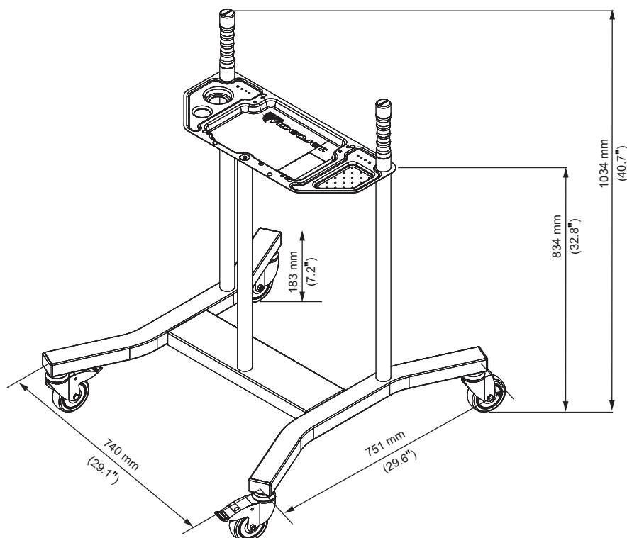
Рис. А-2: Мобильная подставка для принтера
