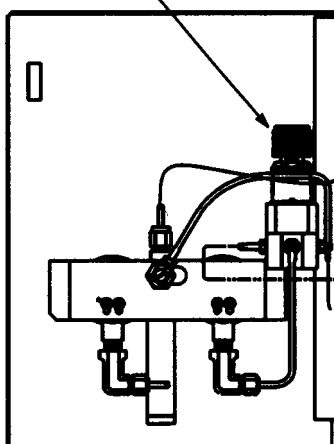
Регулятор давления чернил
