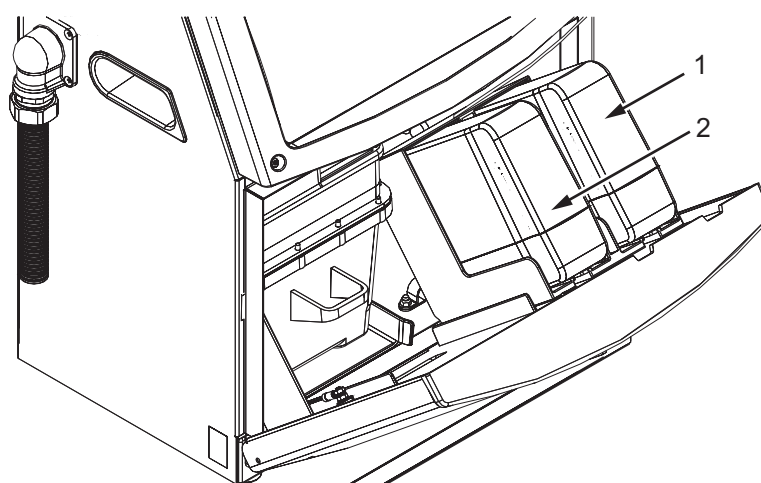
Рис. 6-1: Картриджи со встроенной микросхемой
