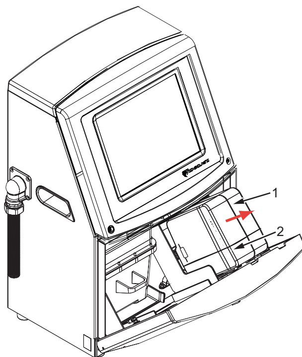
Рис. 6-2: Выемка картриджей
