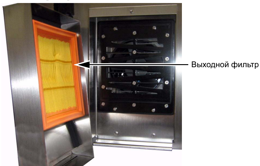
Рис. 3-10: Выходной фильтр (модель IP65)
