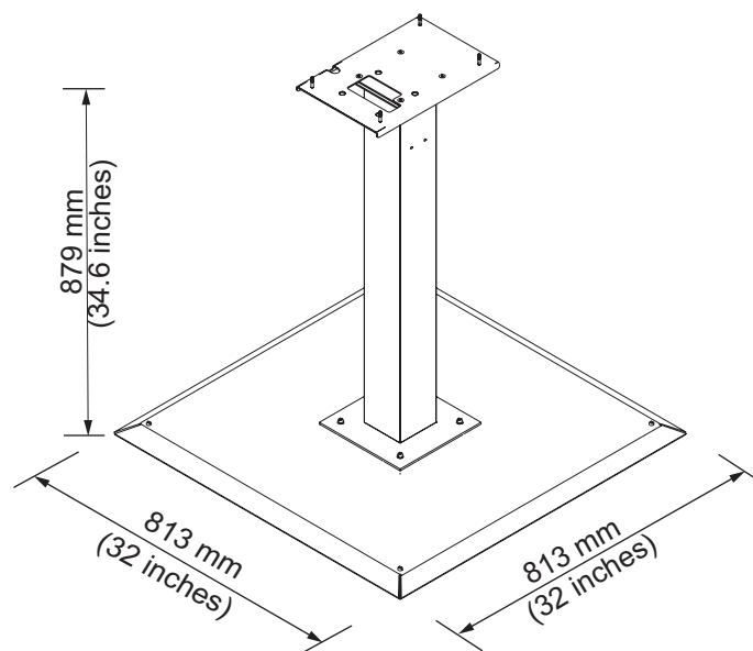
Рис. А-3: Подставка для стационарного принтера
