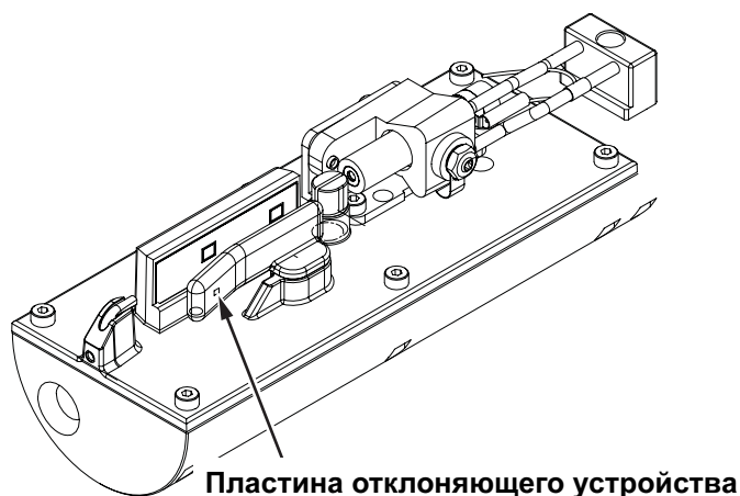
Рис. 6-6: Проведите очистку пластины отклоняющего устройства
