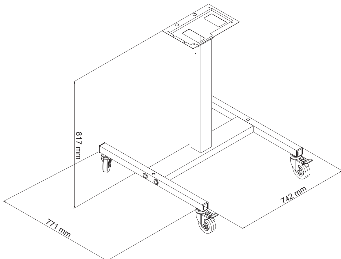
Рис. А-2: Размеры подставки для мобильного принтера
