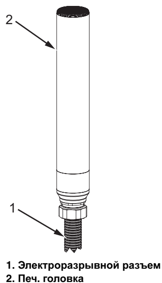
Рис. 3-6: Печатающая головка и электроразрывной разъем
