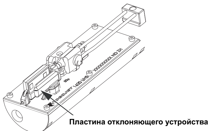
Рис. 6-7: Проведите очистку пластины отклоняющего устройства (Videojet 1650 UHS)
