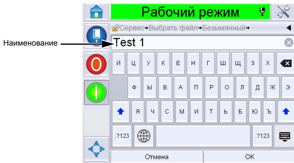
Рис. 5-38: Сохранение сообщения
