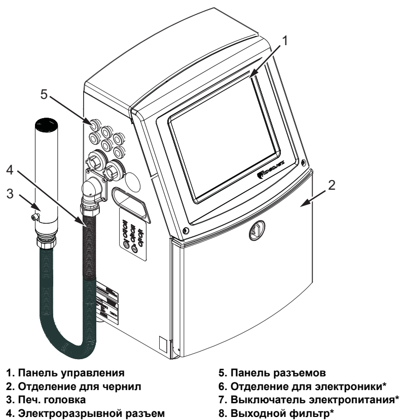
Рис. 3-1: Основные компоненты принтера
