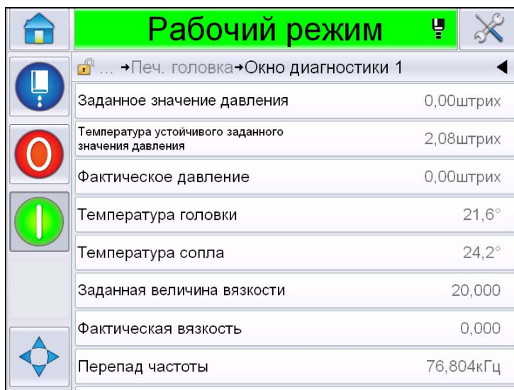
Рис. 5-10: Окно диагностики 1
