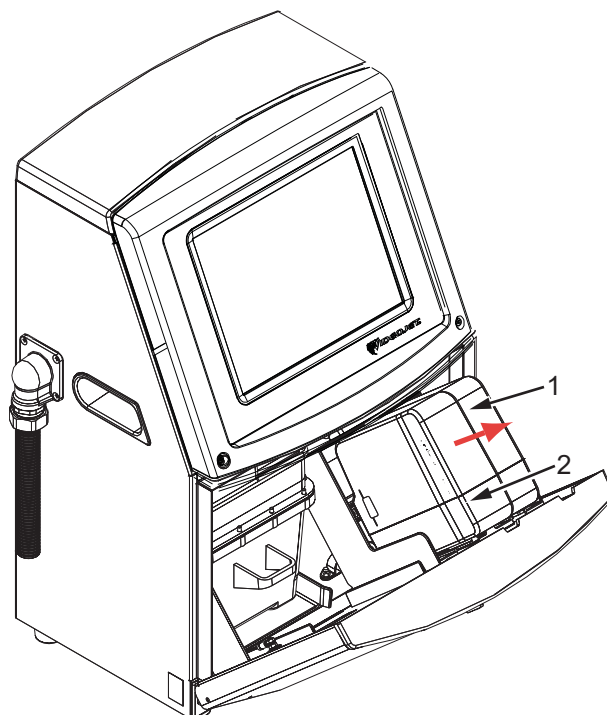
Рис. 6-2: Выемка картриджей
