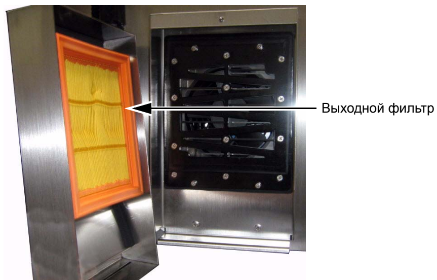
Рис. 3-11: Выходной фильтр (модель IP65)
