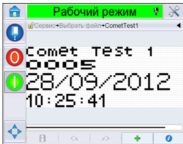
Рис. 5-41: Страница Сообщения
