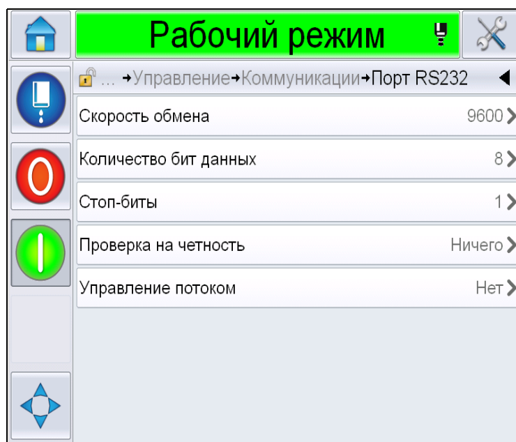
Рис. 4-14: Последовательный порт
