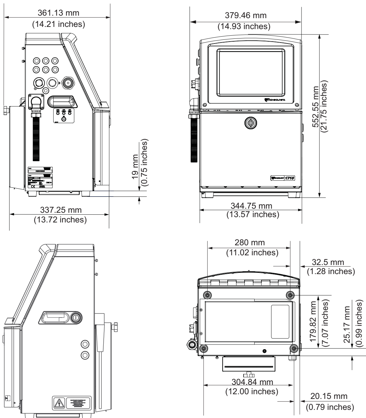
Рис. А-1: Размеры принтера
