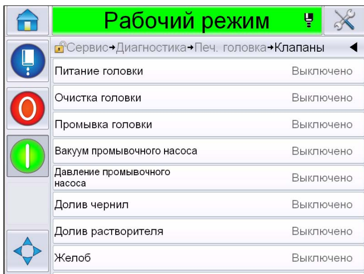
Рис. 5-18: Клапаны
