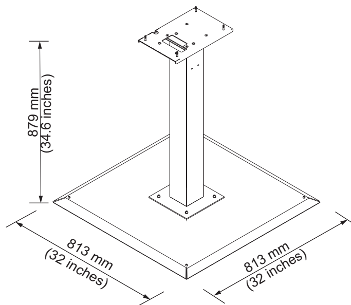
Рис. А-3: Подставка для стационарного принтера
