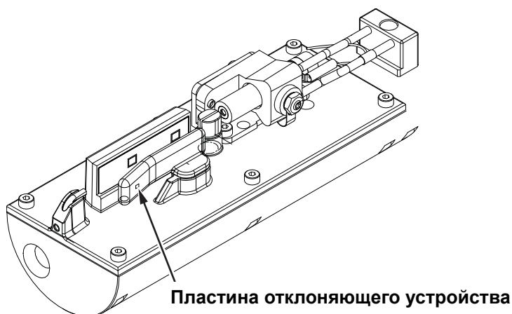
Рис. 6-5: Проведите очистку пластины отклоняющего устройства
