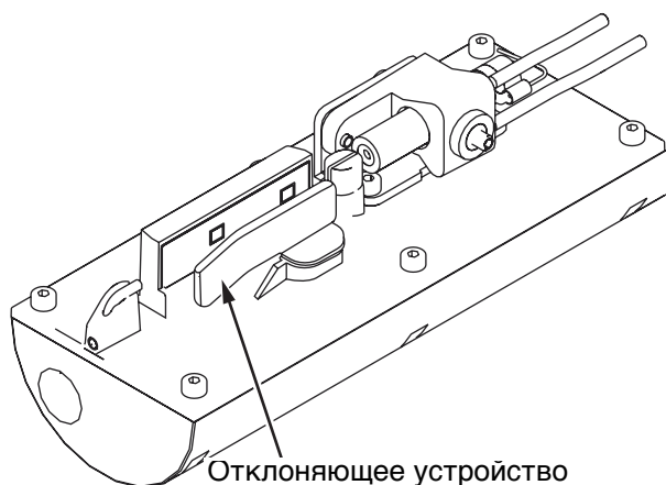
Рисунок 6-5: Проведите очистку пластины отклоняющего устройства
