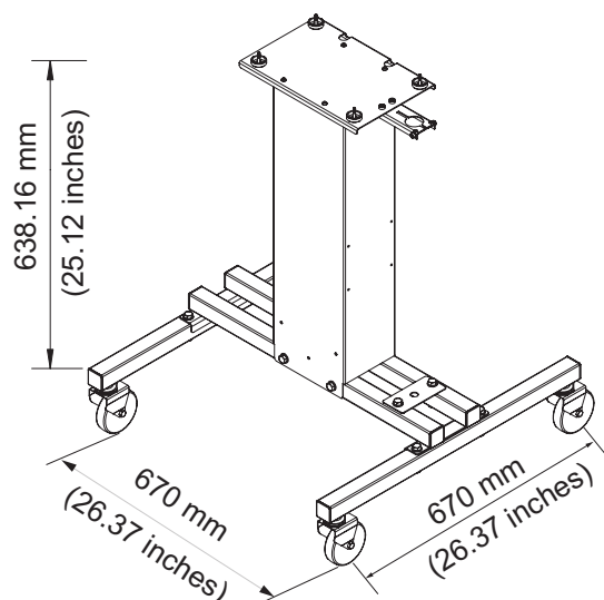
Рисунок А-3: Подставка для мобильного принтера
