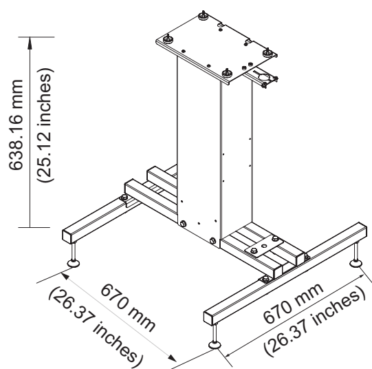
Рисунок А-4: Подставка для стационарного принтера
